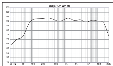
频响特性
