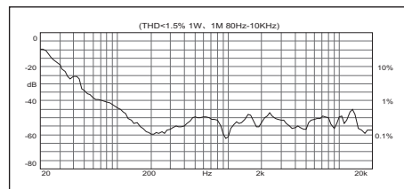
失真特性
