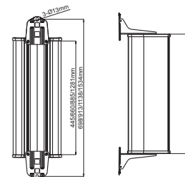
安装示意图
